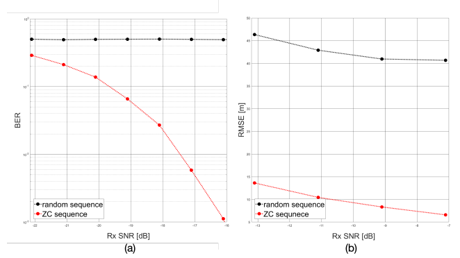
그림 3. 시퀀스 인덱스의 BER(a), 단말 위치의 RMSE(b)
